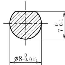
A-A (2:1)
