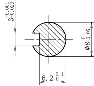
A-A (2:1)
