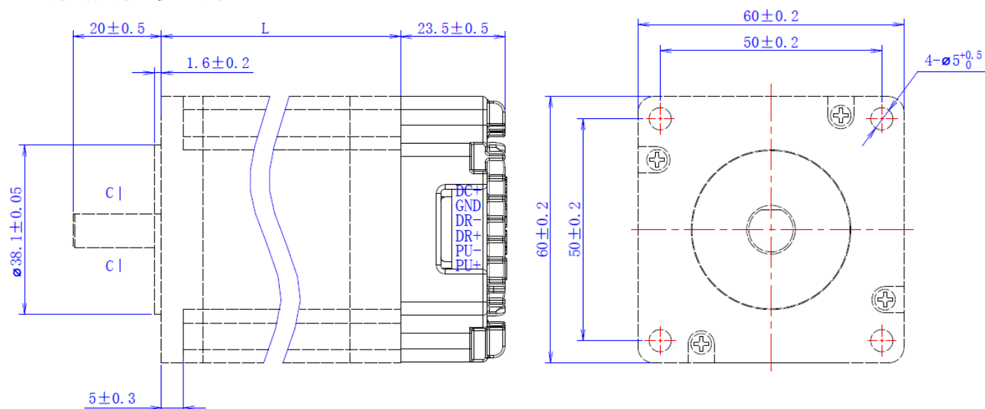
60 一体式步进电机尺寸图
