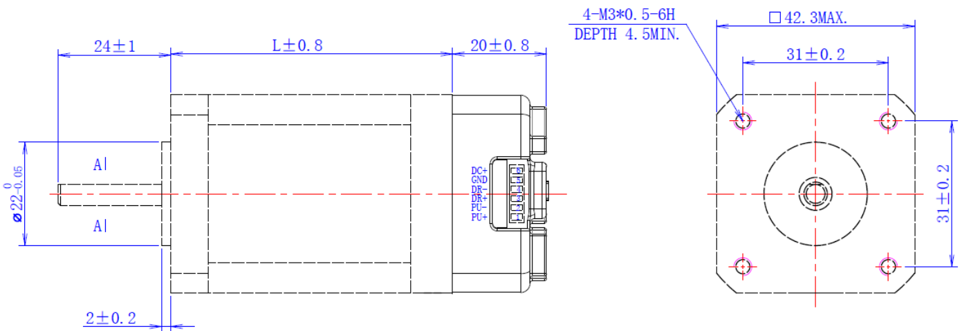
42 一体式步进电机尺寸图
