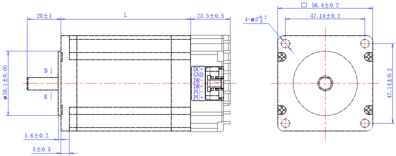
57 一体式步进电机尺寸图
